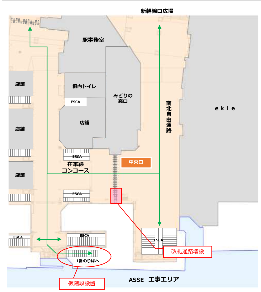
広島駅2F平面図
